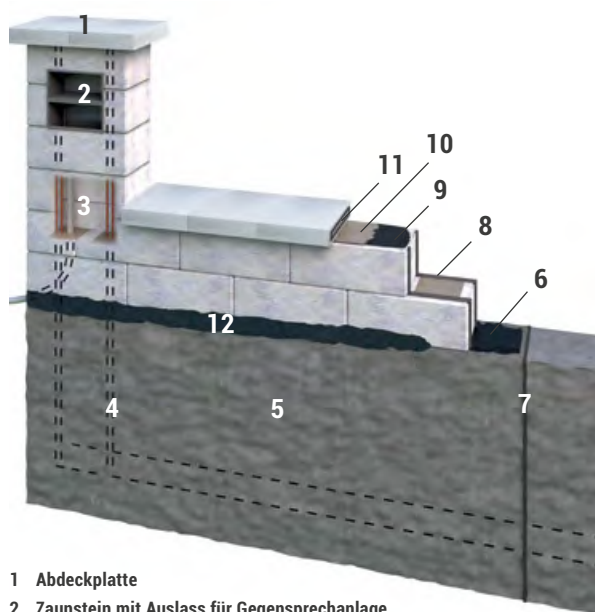
Abbildung 9: Zaunaufbau
